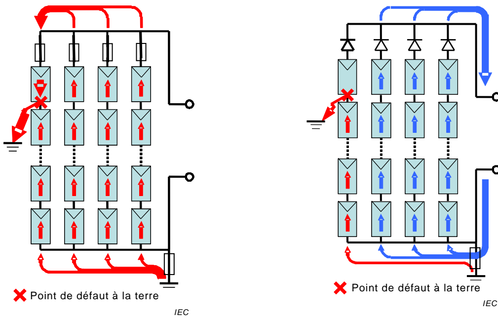
a) Sans diode antiretour
