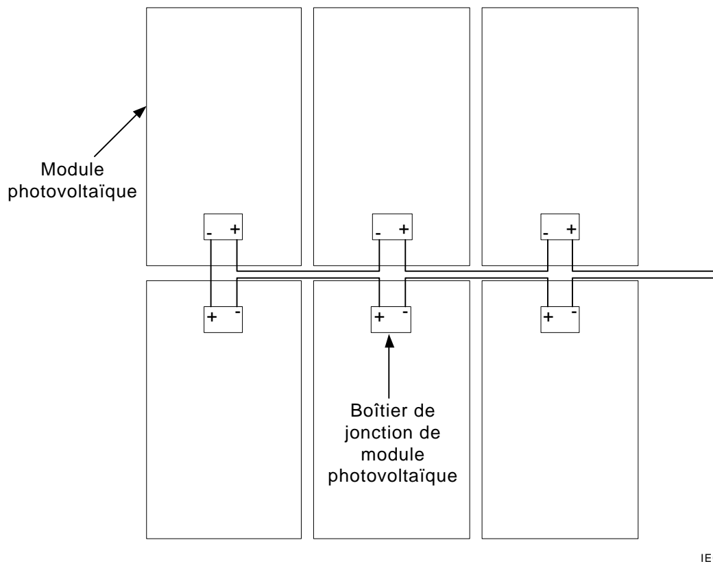
Figure 12 b) - Câblage surface de boucle minimum exemple 2
