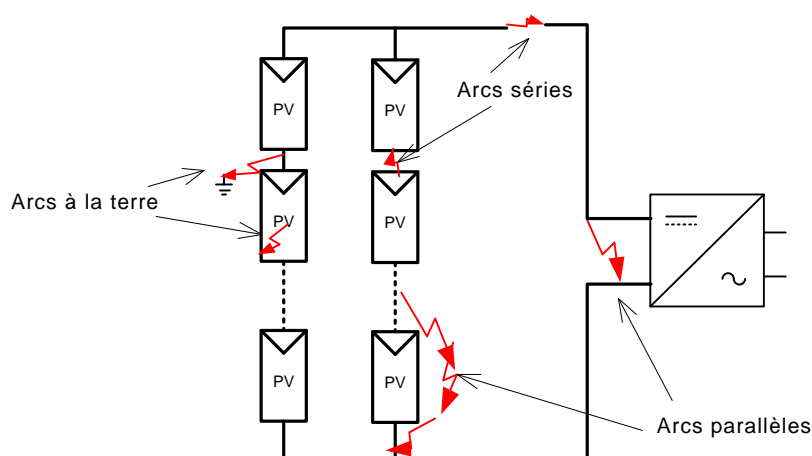
Figure D.1 – Exemples de types d'arcs dans les groupes photovoltaïques
