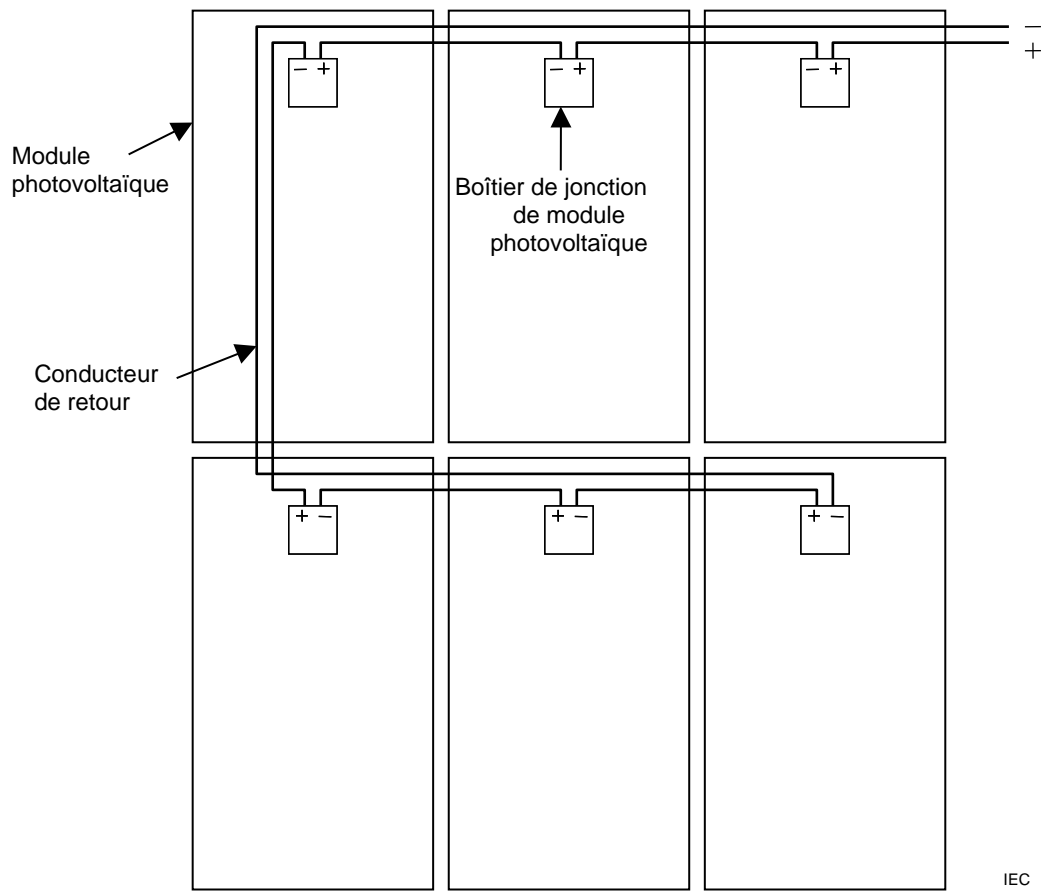
Figure 12 a) - Câblage surface de boucle minimum exemple 1
