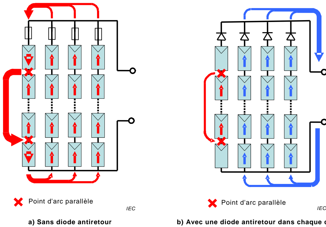
Figure C.1 – Effet d'une diode antiretour en cas de court-circuit dans une chaîne photovoltaïque
