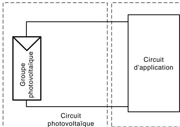
Figure 1 – Configuration fonctionnelle générale d'un système photovoltaïque
