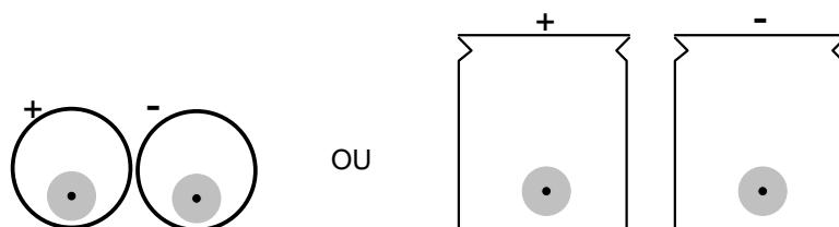
Figure 9b – Câble à un conducteur, dans un conduit ou une goulotte isolé(e) approprié(e)
