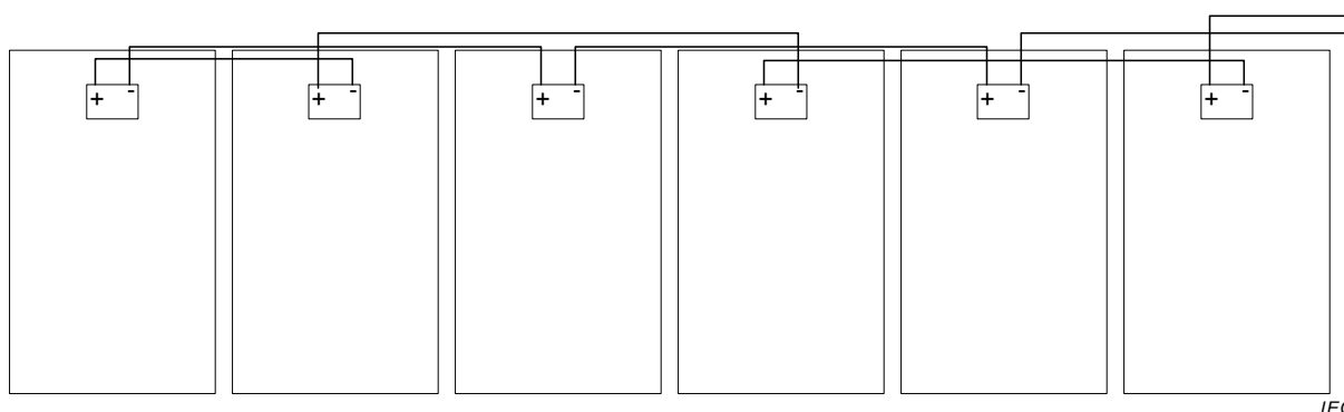
Figure 12 c) – Câblage surface de boucle minimum exemple 3
