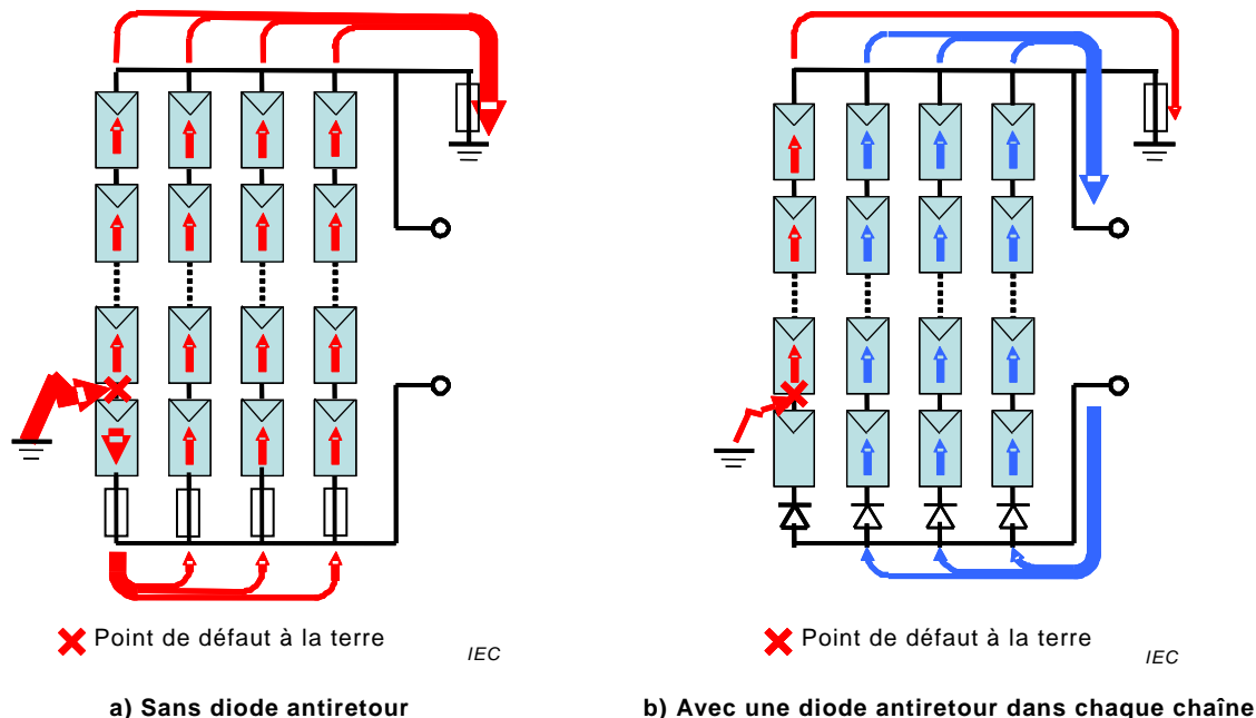
Figure C.3 – Effet d'une diode antiretour en cas de défaut à la terre sur un système avec mise à la terre du côté positif
